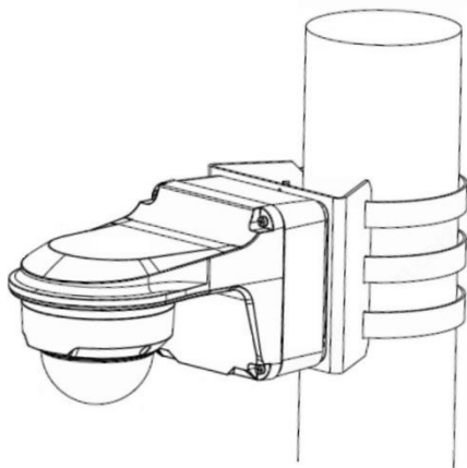
壁面取付金具 + ポール取付金具 TR-JB07/WM03-G-IN + TR-UP06-IN
